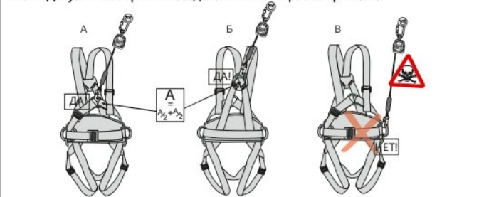
Рис. 4. Допустимые варианты соединения «НВ-02 трос» с привязью
