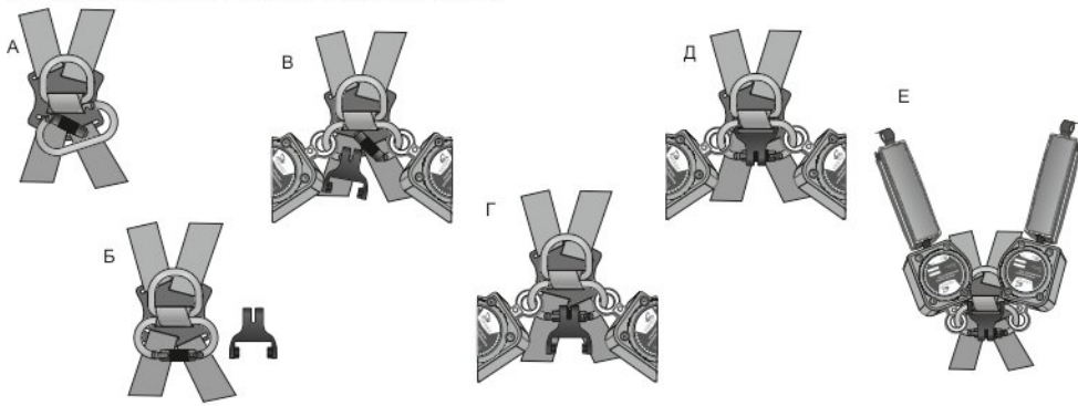
Рис. 9. Установка адаптера на двухплечевой «НВ-02 трос»
