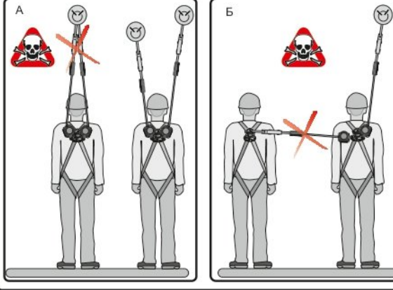
Рис. 12. Ограничения использования двухплечевого «НВ-02 трос»
